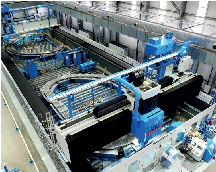
Fraiseuse double portique (X 30000, Y 9000, Z 1250 mm, charge max. : 5 tonnes / m 2 ).
