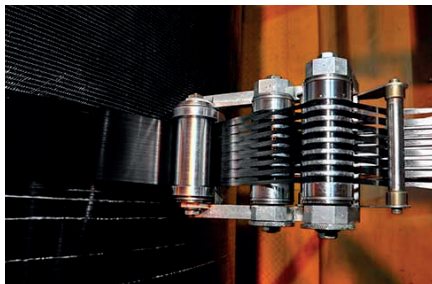
Enroulement filamentaire.
