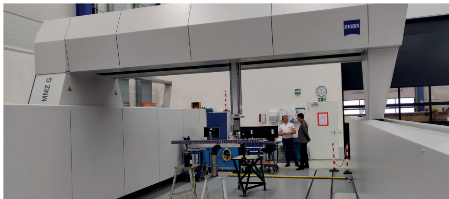
Contrôler au 10 ème de millimètre près avec la machine ZEISS MMZ-G. ( X 4000 Y 8000 Z 2000 mm).
