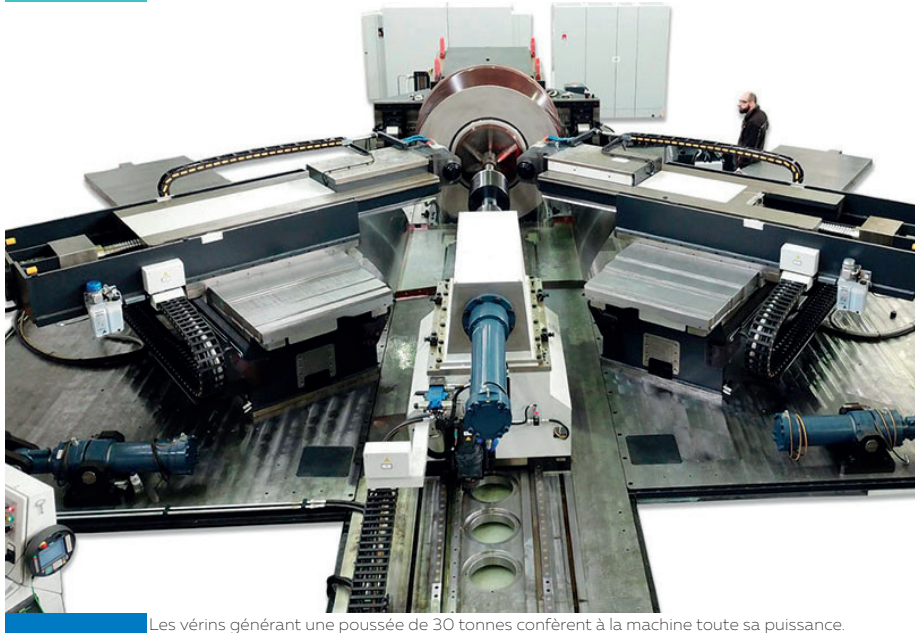
Les vérins générant une poussée de 30 tonnes confèrent à la machine toute sa puissance.
