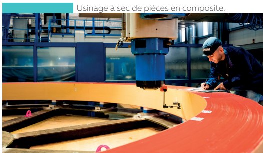
Usinage à sec de pièces en composite.
