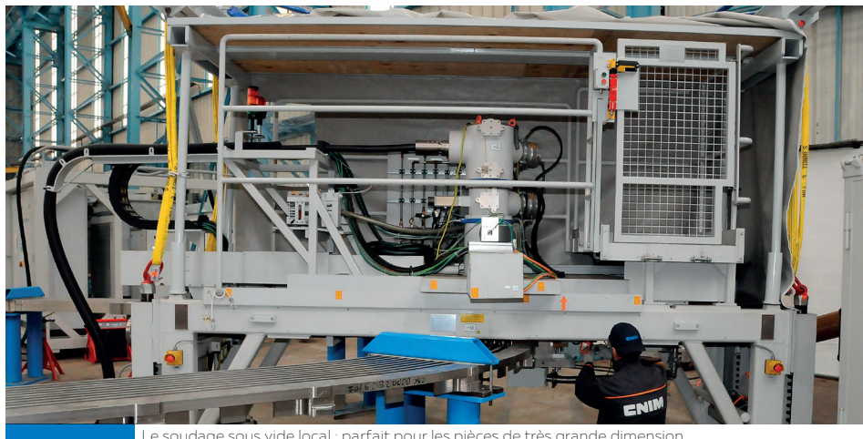
Le soudage sous vide local : parfait pour les pièces de très grande dimension.
