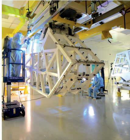
Les assemblages les plus complexes et exigeants sont réalisés en salle blanche ISO 6.
